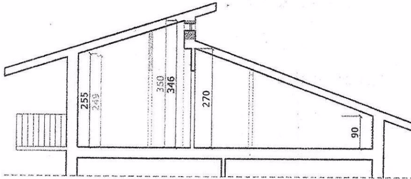
SEZIONE A-A' - STATO DI CONFRONTO
