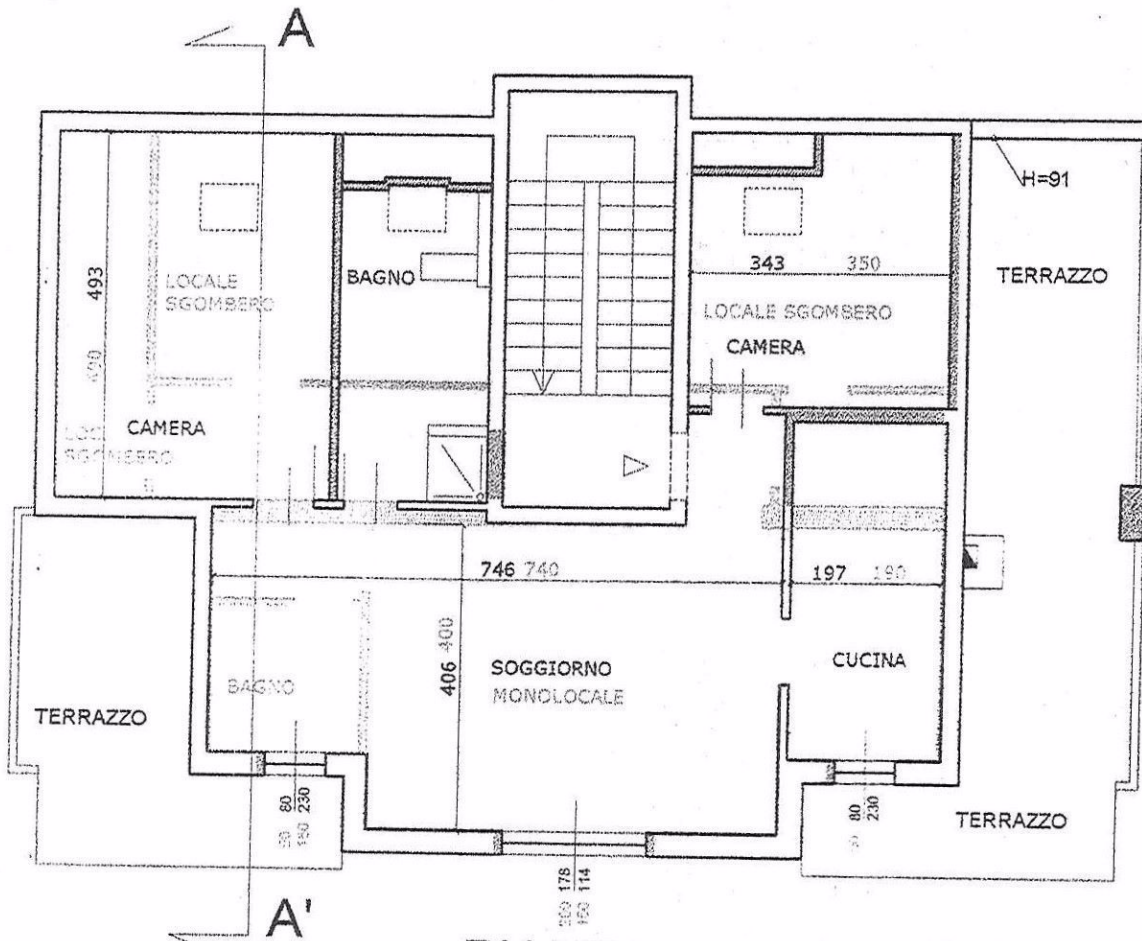
PIANTA STATO DI FATTO
