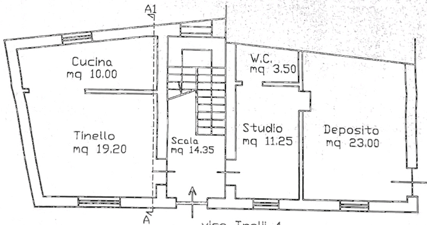
PIANO TERRA h=3.10
