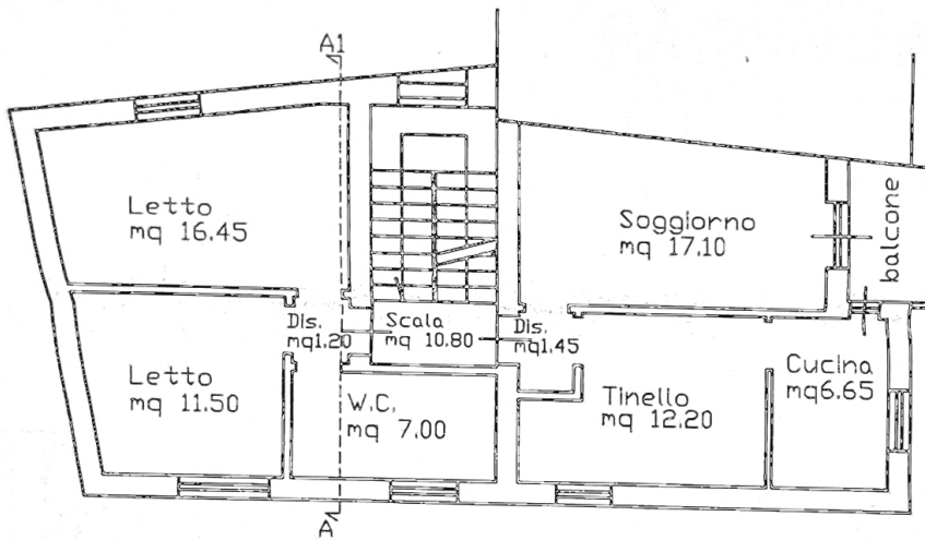
PIANO PRIMO h=3.00
