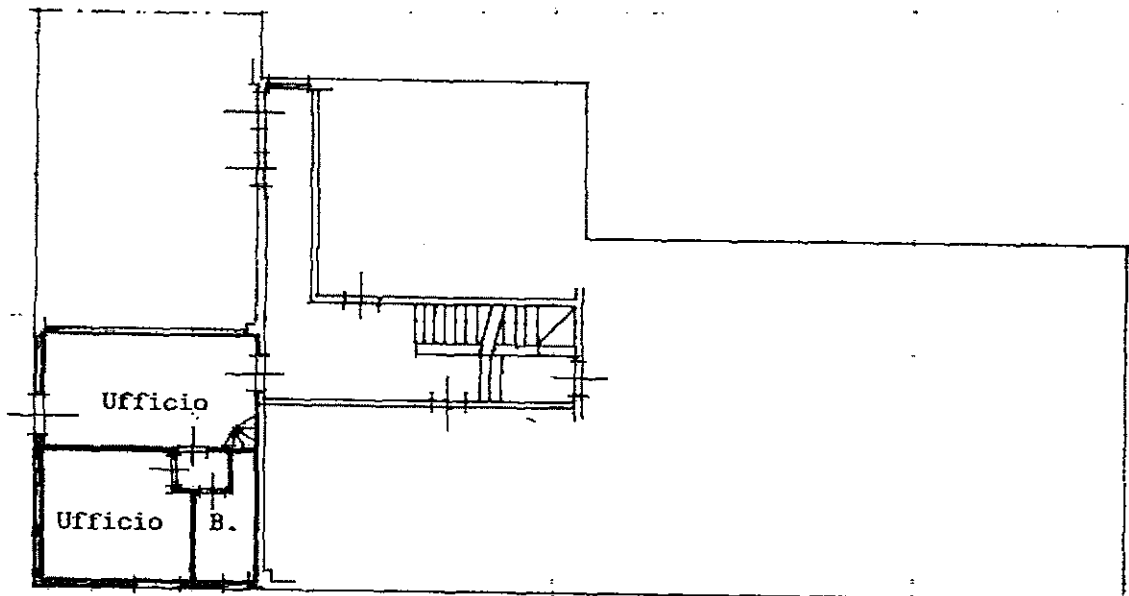
PIANO PRIMO H= 2.70
