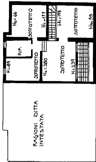
SOTTOTETTO
