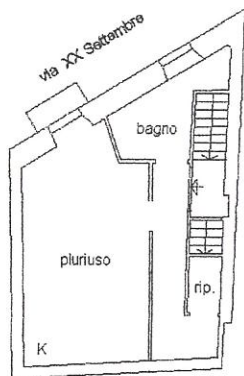
PIANO PRIMO h=2,80
