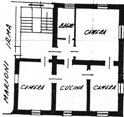
PIANO SECONDO H = 3.0 m
