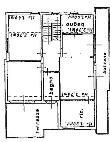
PIANO SECONDO h = 2.70
